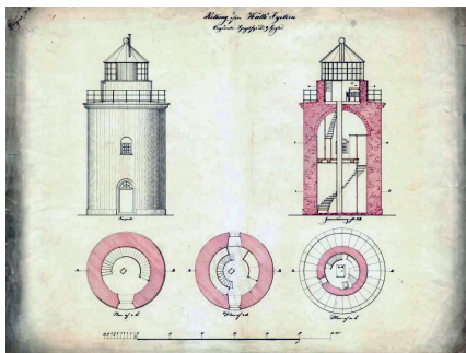
Hällö fyr 1842.
