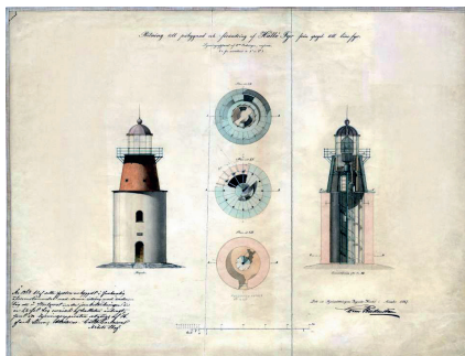
Hällö fyr 1868.
